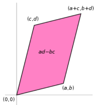
Figure 1.1: Interpretación geométrica del determinante
